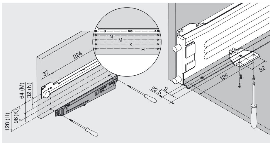
Süsteem 32: BLUMOTIONi kokkupanekul kasutatakse 32 mm puurimissüsteemi.
